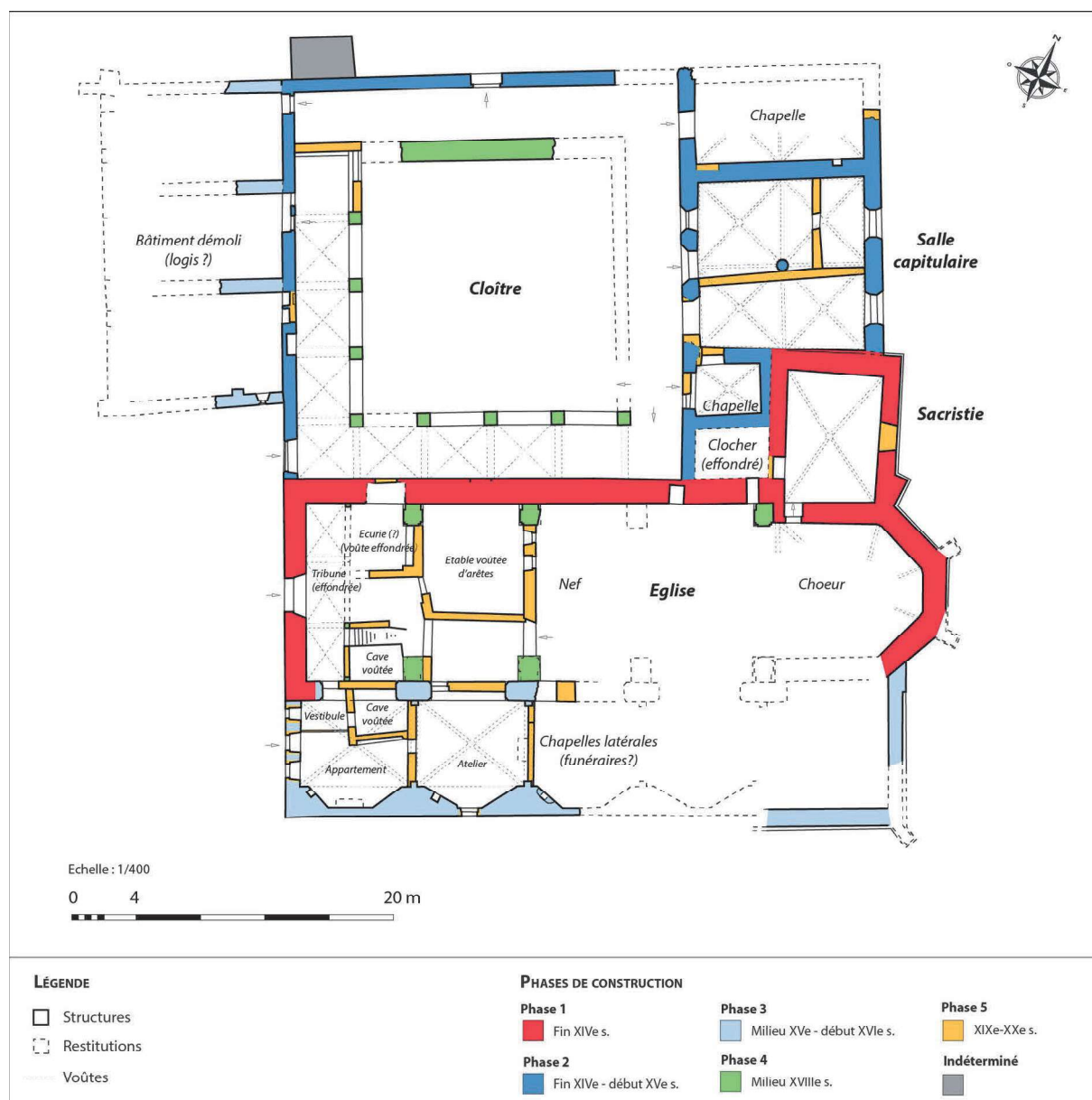
Figure 3 : Couvent des cordeliers de La Chambre, phases de construction. Dessin : E. Chauvin-Desfleurs, L. D'Agostino, 2021.
