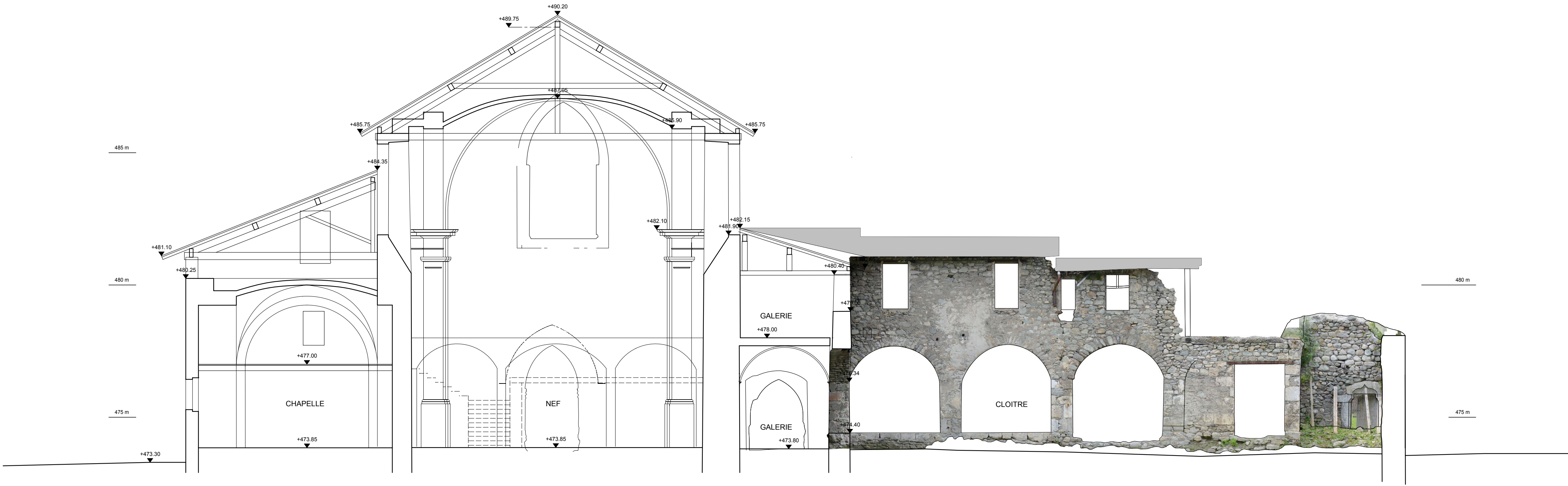
coupe BB'
